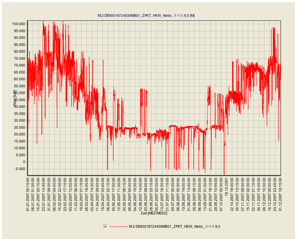
2007_Lastverlauf Einspeisung 60 kV:
